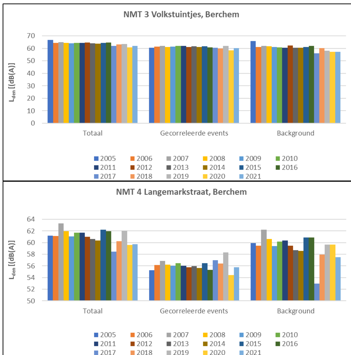
Figuur 14: Evolutie van de geluidsbelasting op basis van L_{den} gedurende voor de jaren 2005 tot en met 2021
