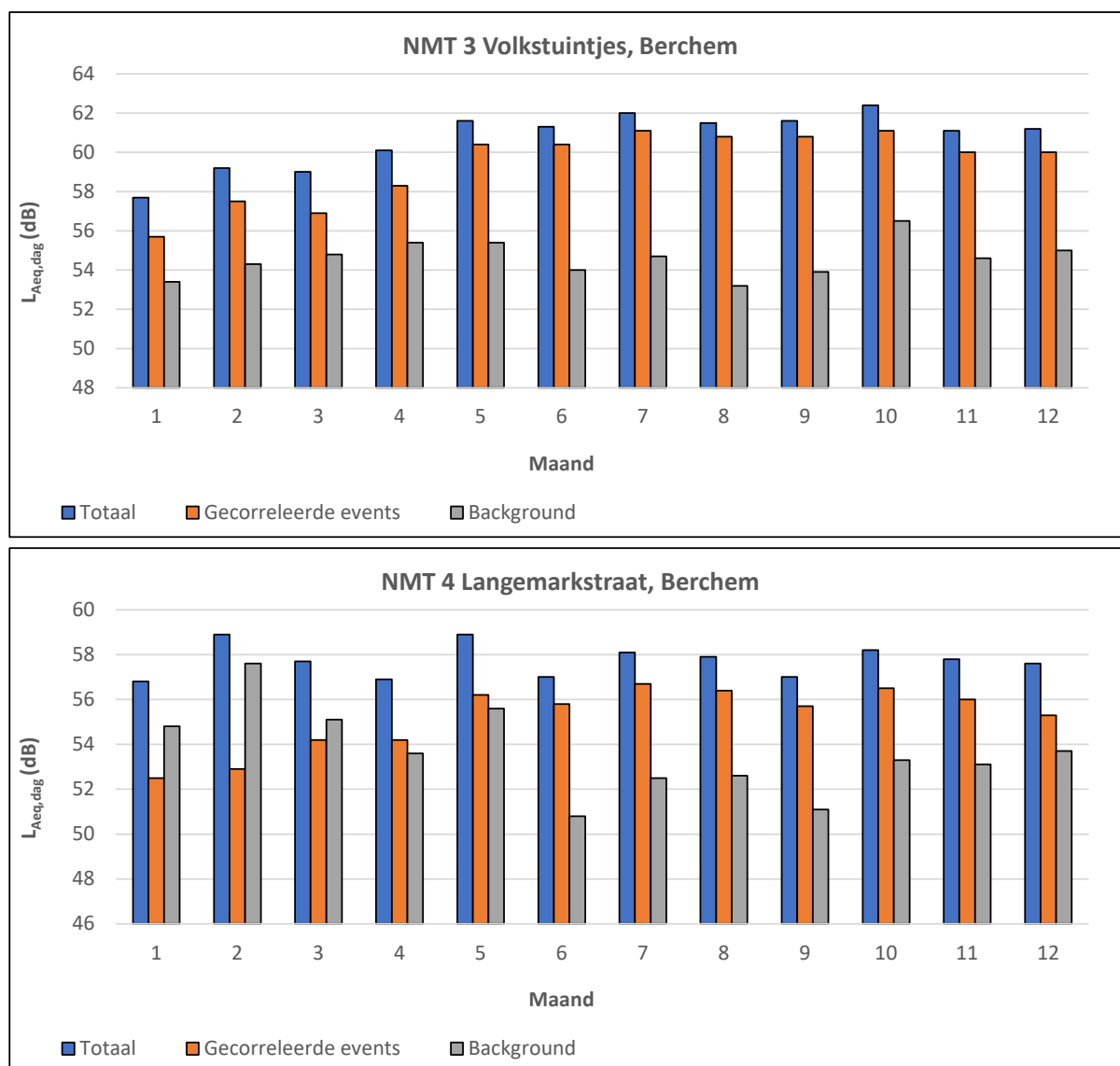
Figuur 7: Analyse per maand van de gemeten equivalente geluidsdruk niveaus op basis van de voor oude VLAREM geldende uurregeling (dag: 06u00 – 23u00, nacht: 23u00-6u00)
