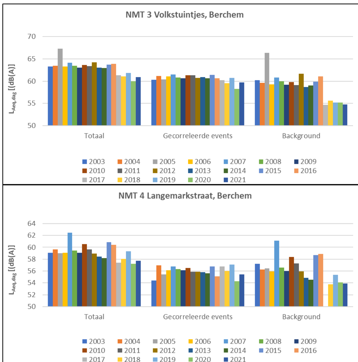
Figuur 13: Evolutie van de geluidsbelasting op basis van L_{Aeq} gedurende de dag-periode (dag: 06u00 – 23u00) voor de jaren 2003 tot en met 2021
