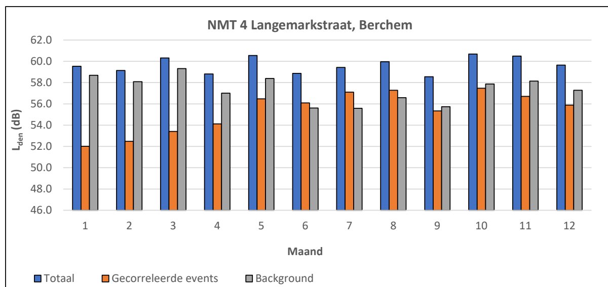
Figuur 8: Analyse per maand van de gemeten L_{den} -niveaus overeenkomstig de uurregeling van de nieuwe VLAREM-wetgeving (cfr. EU-richtlijn).
