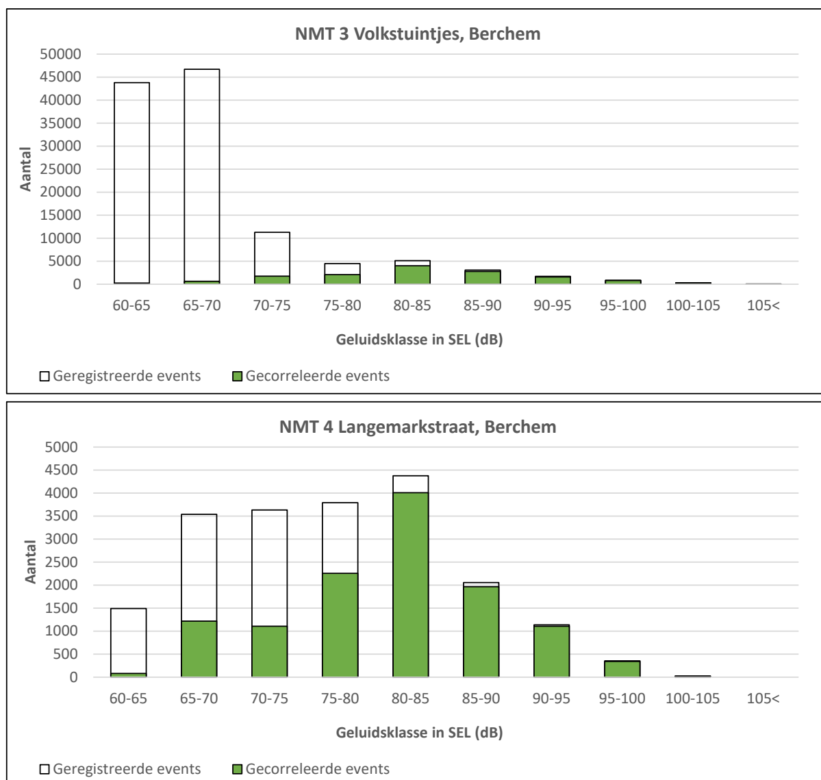
Figuur 5: Statistische analyse van de geluidsgebeurtenissen op basis van SEL-klassen van 5 dB(A)
