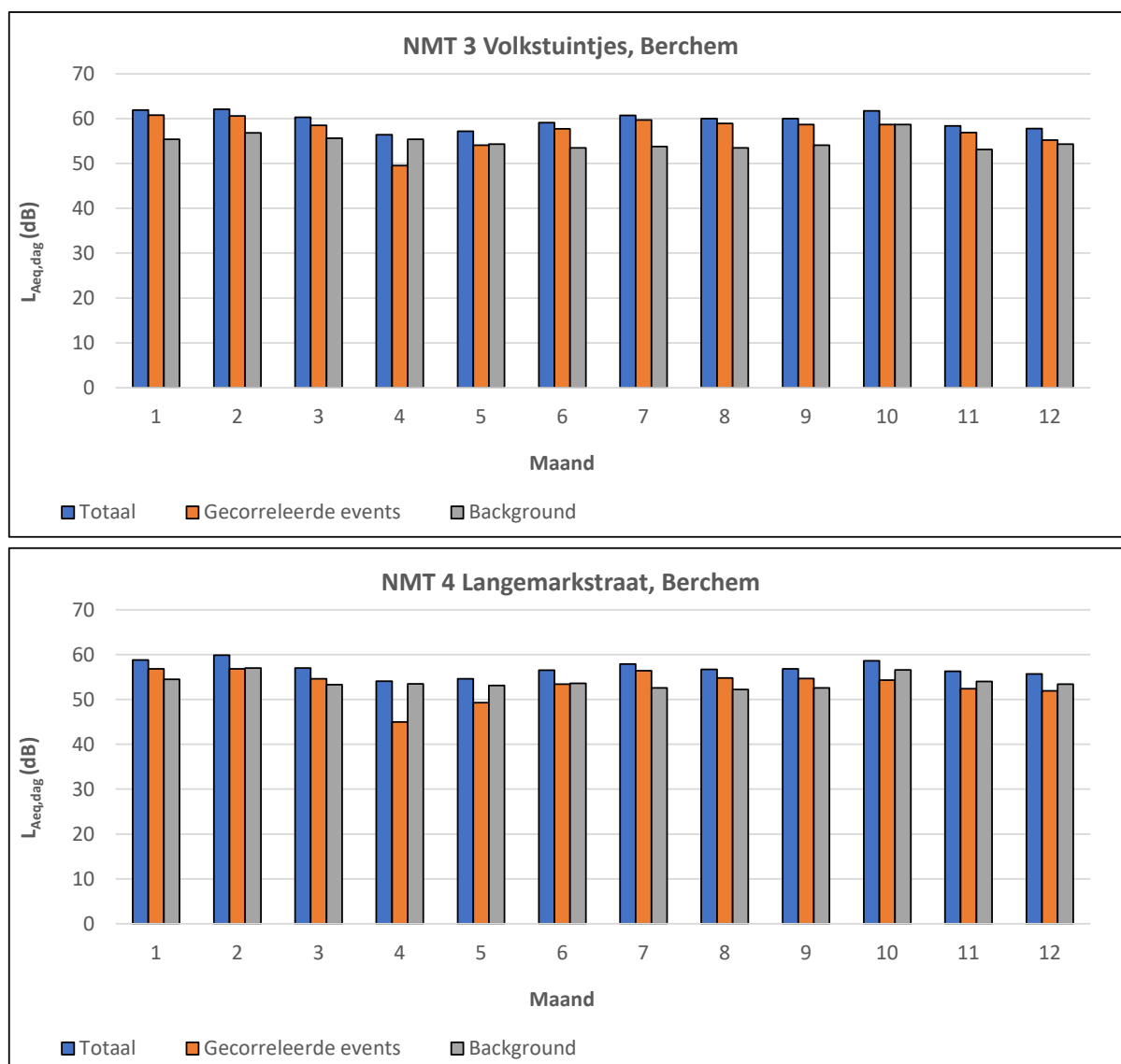
Figuur 7: Analyse per maand van de gemeten equivalente geluidsdrukkniveaus op basis van de voor oude VLAREM geldende uurregeling (dag: 06u00 – 23u00, nacht: 23u00-6u00)
