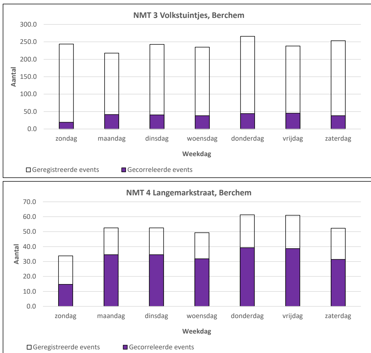
Figuur 3: Analyse van het gemiddeld aantal geluidsgebeurtenissen per weekdag (dag : 06u30 – 23u00)
