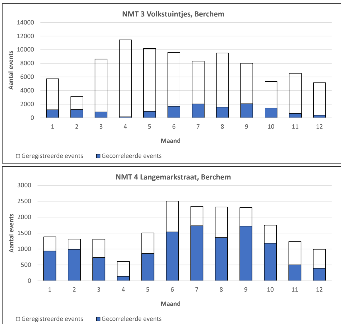
Figuur 2: Analyse van het aantal geluidsgebeurtenissen per maand tijdens de openingsuren van de luchthaven (dag : 06u30 – 23u00)
