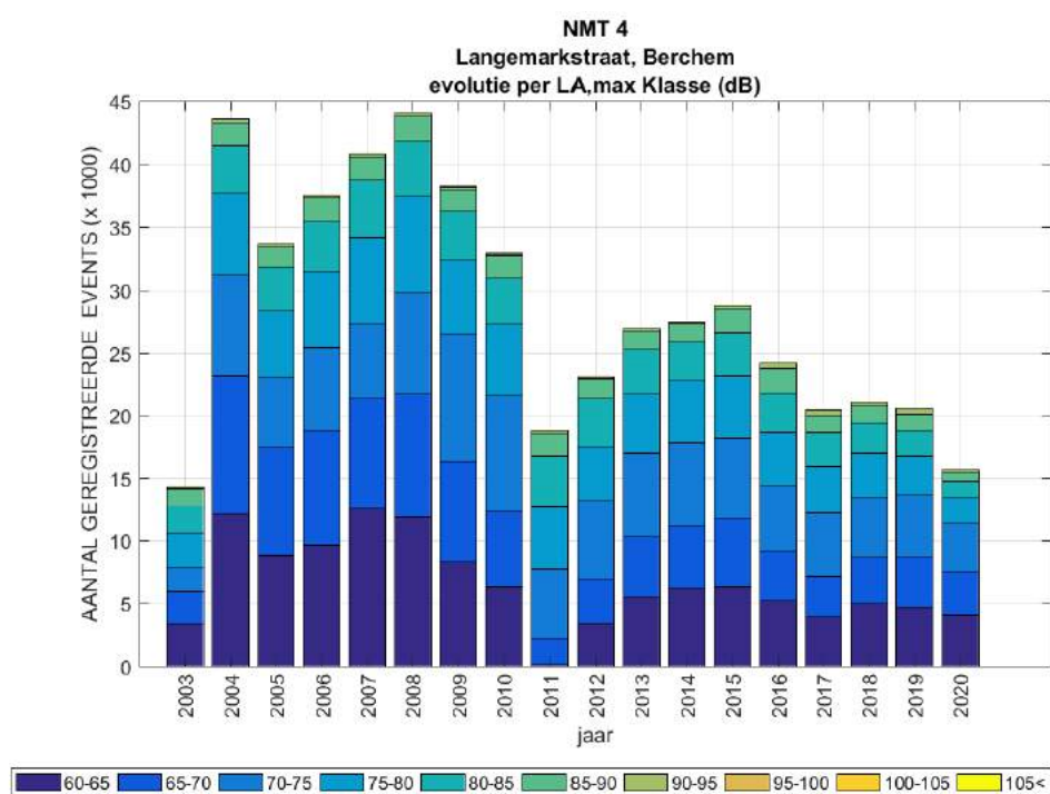
Figuur 11: Evolutie van het totaal aantal geregistreerde geluidsgebeurtenissen op basis van L_{Amax} -klassen van 5 dB(A) voor de jaren 2003 tot en met 2020
