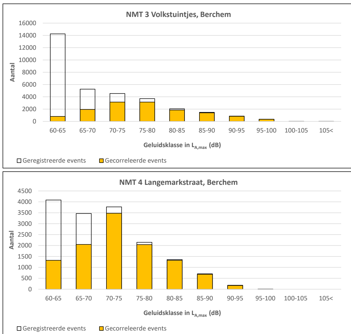
Figuur 6: Statistische analyse van de geluidsgebeurtenissen op basis van L_{A,max} -klassen van 5 dB(A)
