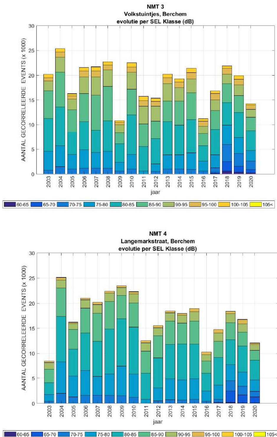
Figuur 10: Evolutie van het totaal aantal gecorreleerde geluidsgebeurtenissen op basis van SEL-klassen van 5 dB(A) voor de jaren 2003 tot en met 2020
