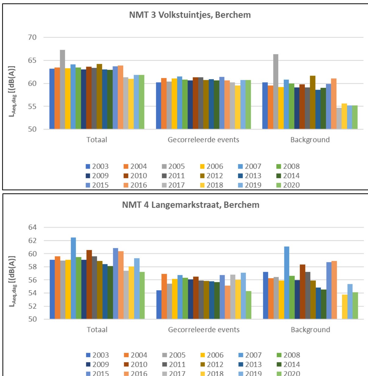
Figuur 13: Evolutie van de geluidsbelasting op basis van L_{Aeq} gedurende de dag-periode (dag: 06u00 – 23u00) voor de jaren 2003 tot en met 2020
