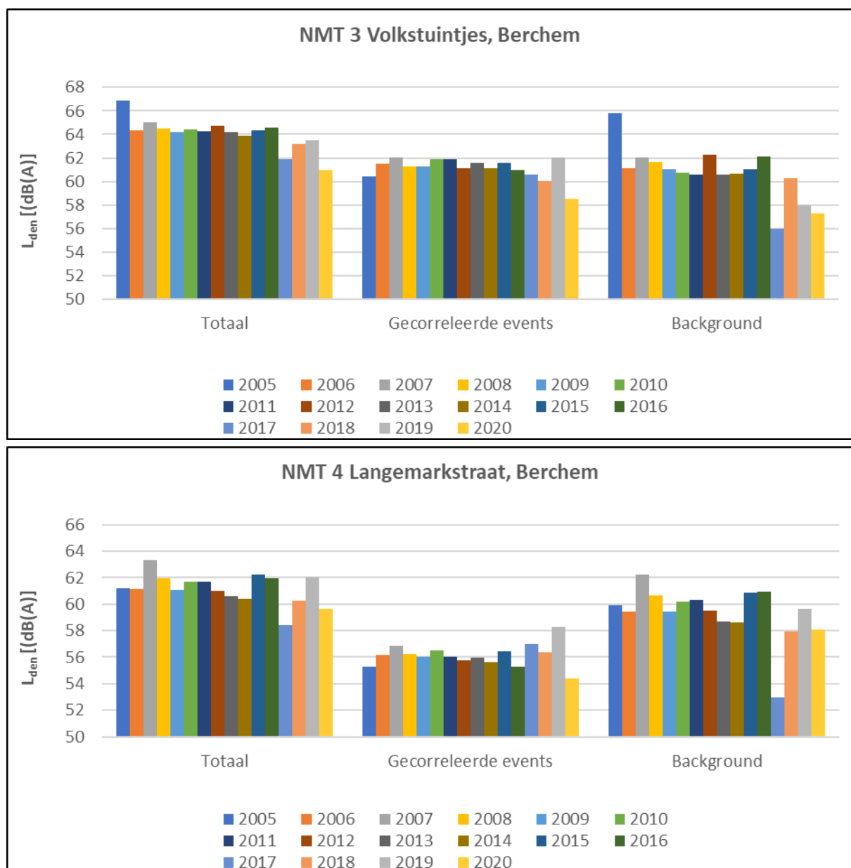
Figuur 14: Evolutie van de geluidsbelasting op basis van L_{den} gedurende voor de jaren 2005 tot en met 2020
